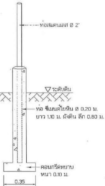
รูปตัด มาตราส่วน 1 : 15
