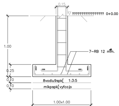
DETAIL F1
