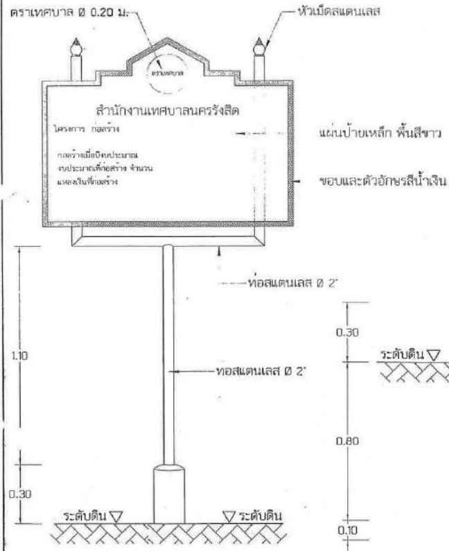
รูปด้าน มาตราส่วน 1 : 15
