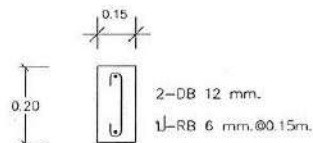
ด้าน B1
