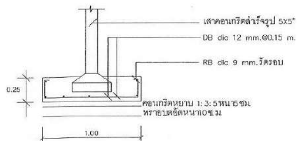
รูปตัด F1
